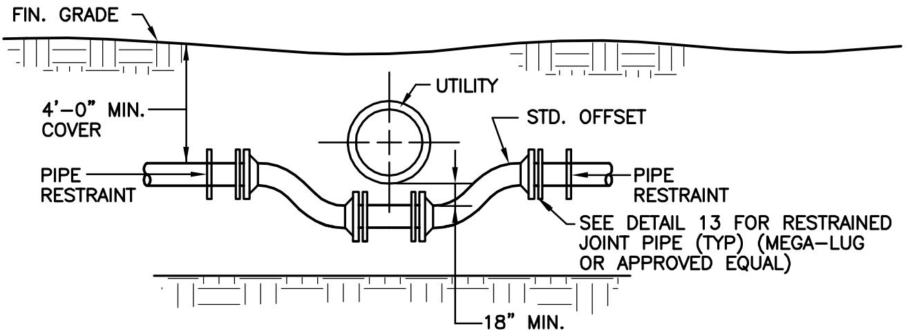
USING STD. OFFSETS
